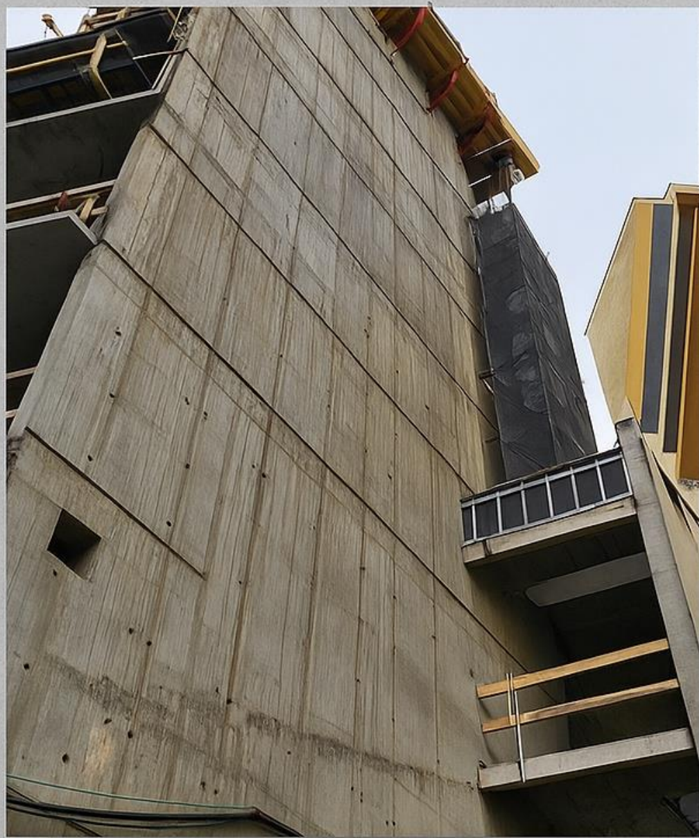
09 | MURO VERTICAL DE EDIFICIO – RECUPERACIÓN INTEGRAL DE HORMIGÓN
